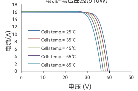
电流-电压曲线(510W)
