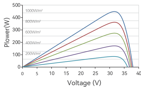
Power-Voltage(450W)
