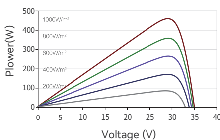
Power-Voltage(455W)
