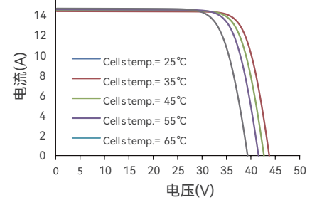
电流-电压曲线(500W)
