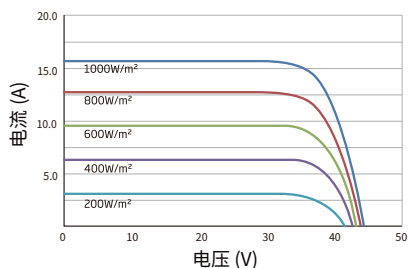
电流-电压曲线 (555W)
