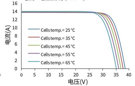
电流-电压曲线 (435W)
