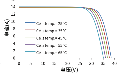
电流-电压曲线 (435W)
