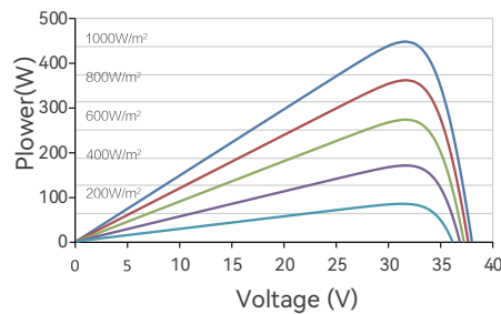
Power-Voltage(450W)
