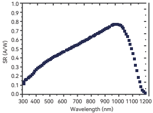
QE曲线
