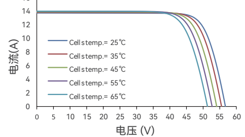
电流-电压曲线(635W)
