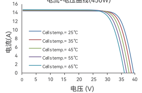
电流-电压曲线(450W)
